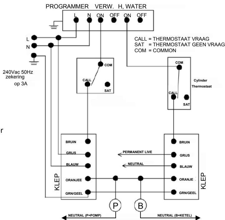
Typisch circuit met twee zone kleppen Z V22 programmeur, kamerthermostaat en boilerthermostaat
